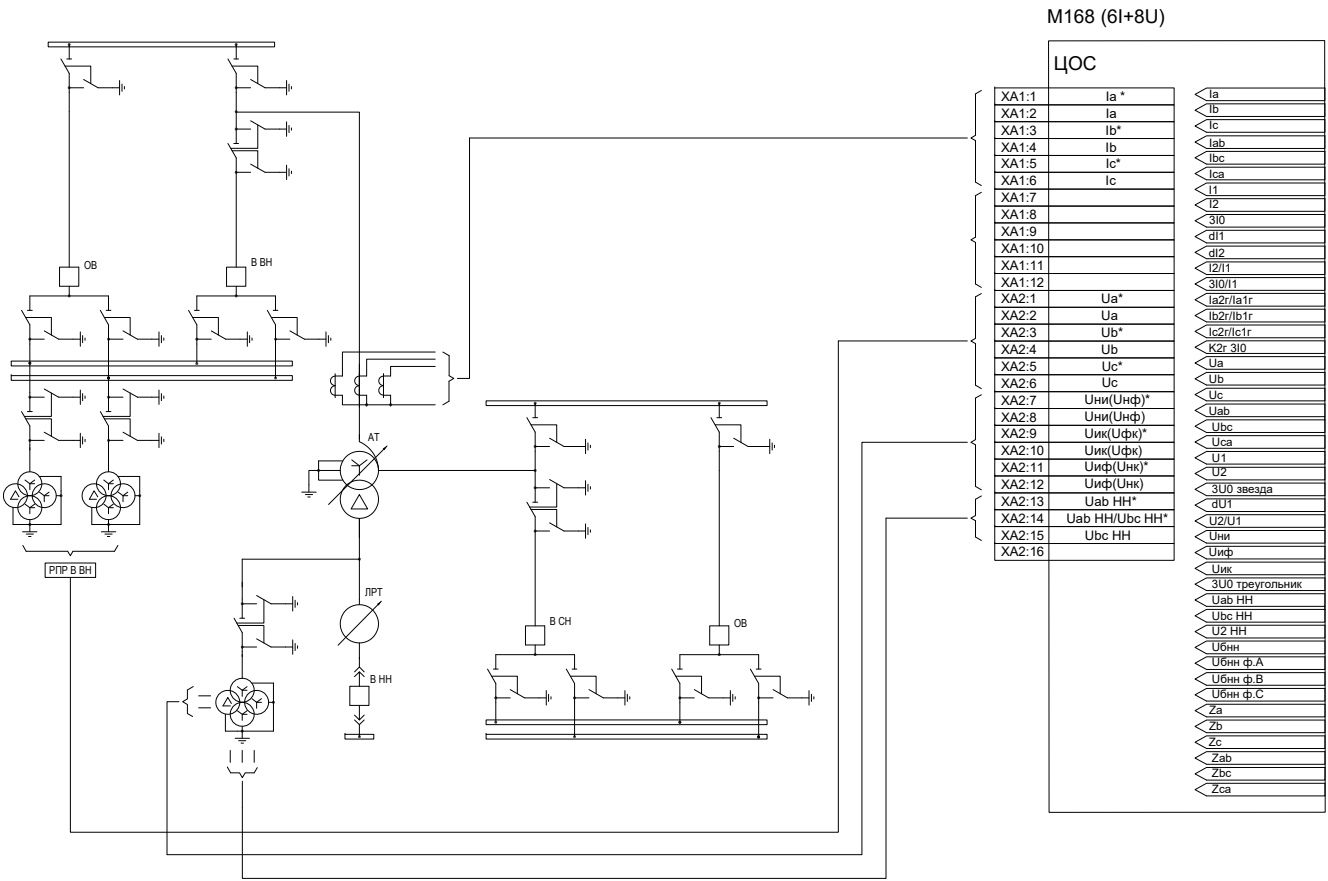
Рисунок Б.1 – Вариант подключения аналоговых цепей ТТ и ТН к устройству
