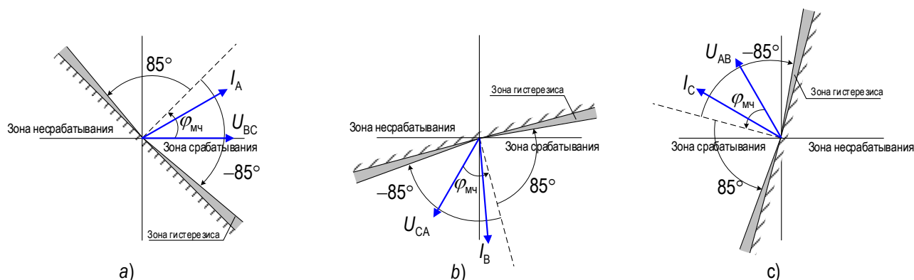
Рисунок 2.26 – Характеристики работы ОНМ:
