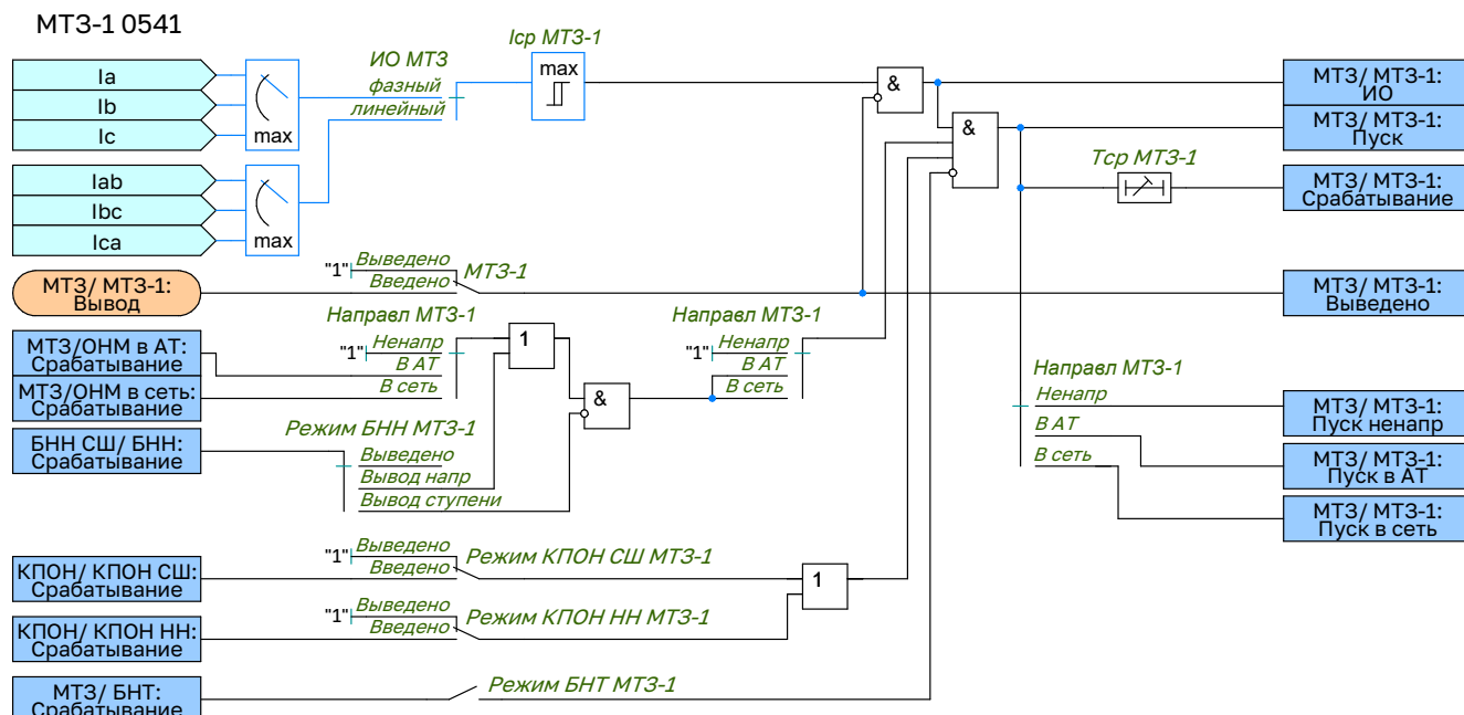
Рисунок 2.23 – Функциональная схема логики МТЗ-1
